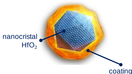
Nanoparticule NBTXR3
